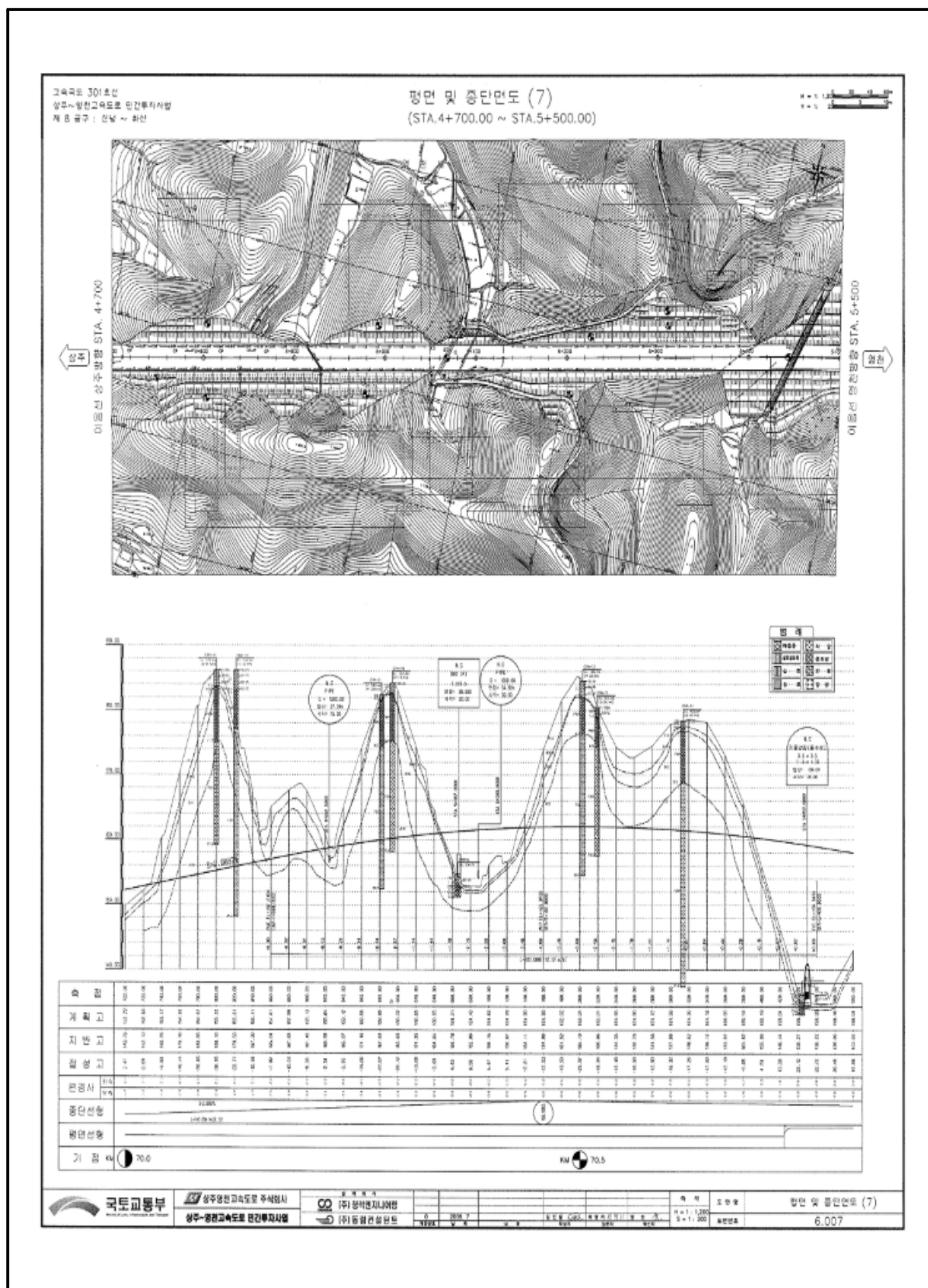
【그림 46.3】 평면도
