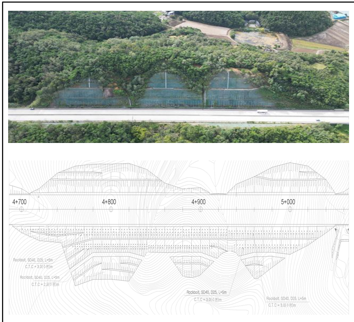
【그림 46.14】 영천절토46 검토대상 비탈면구간
